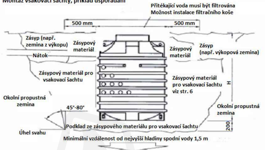
Montáž vsakovací šachty, příklad uspořádání
