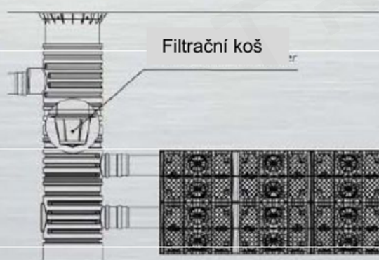
Varianta filtrační šachta
