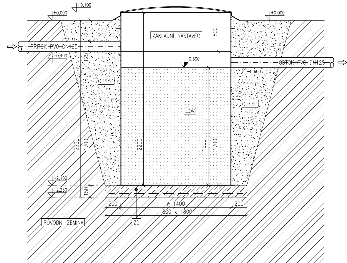
Řez
