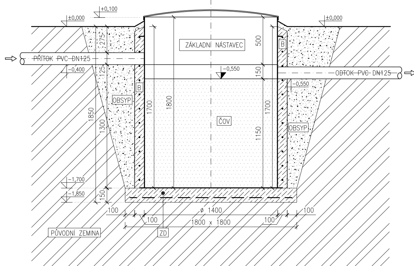
Řez
