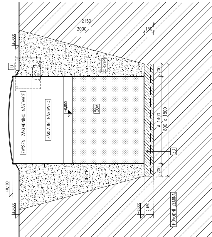
Řez
