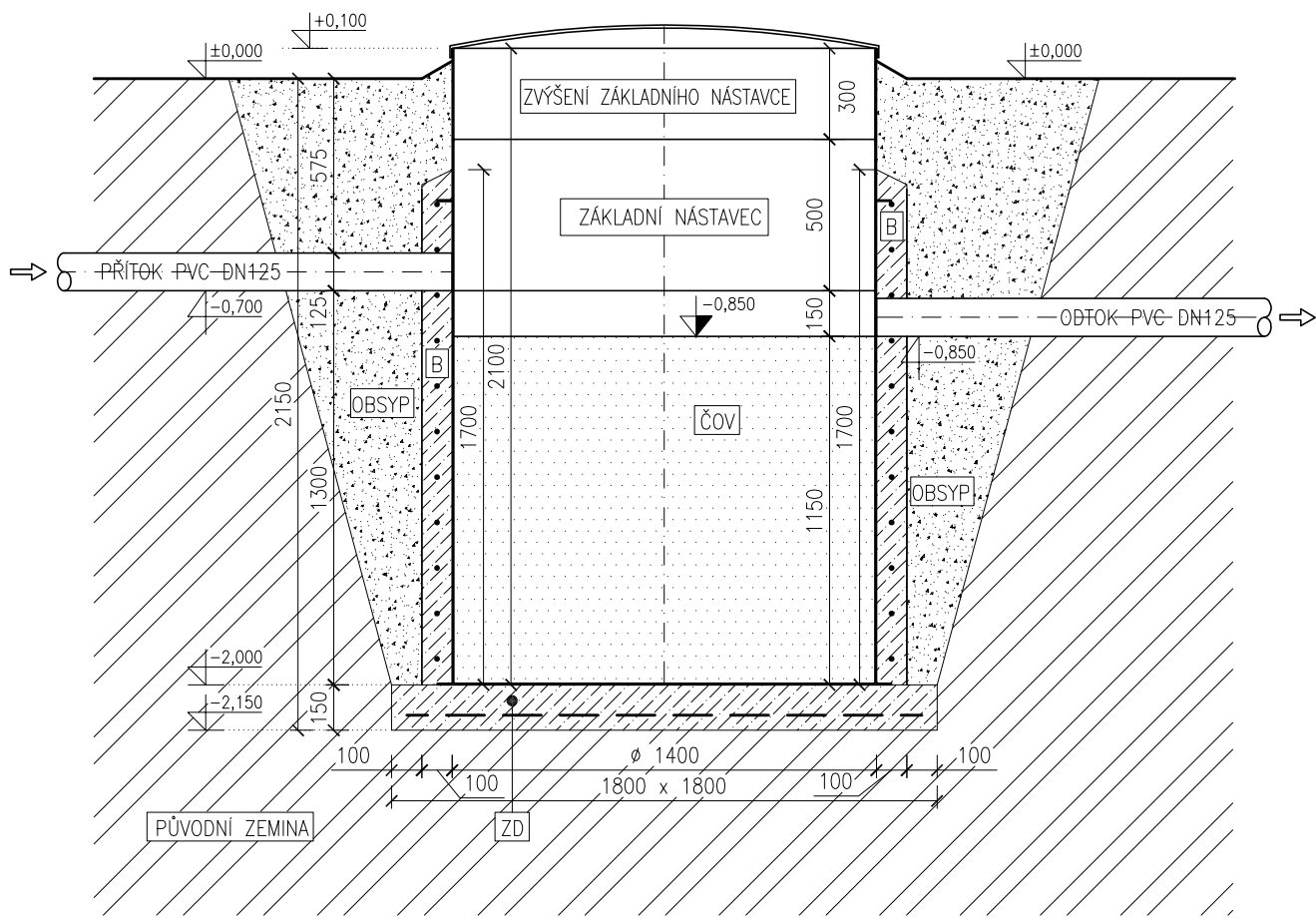
Řez
