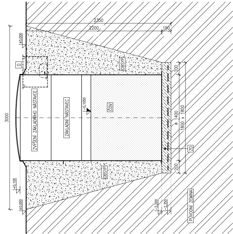
Řez
