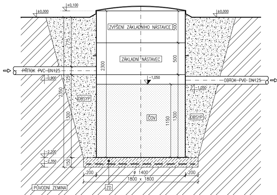
Řez
