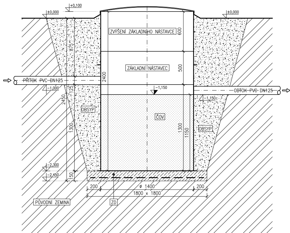
Řez
