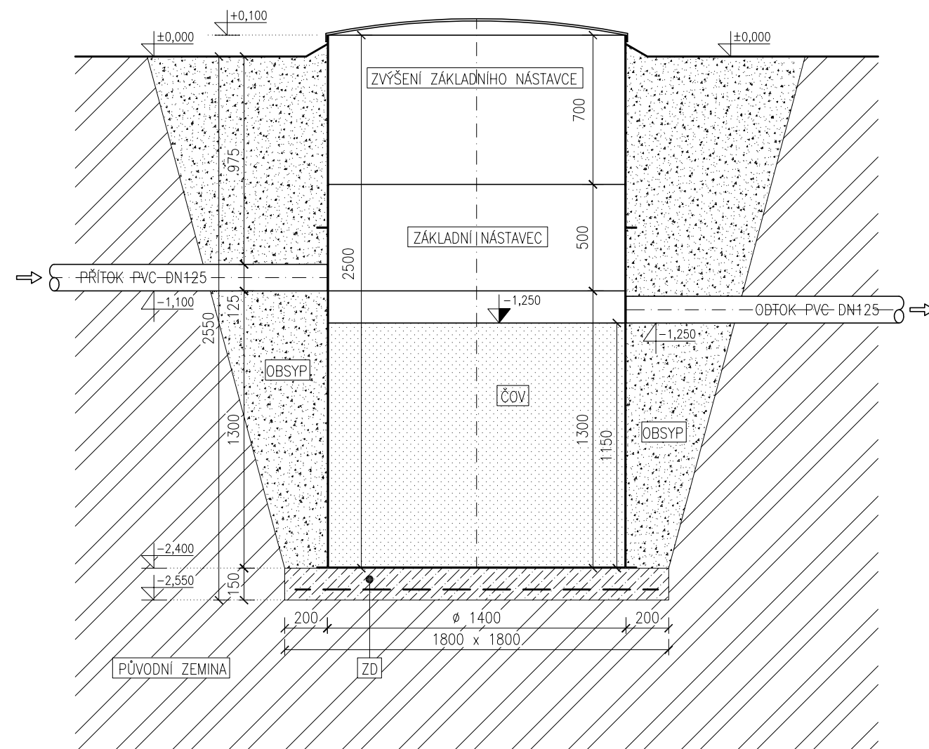
Řez
