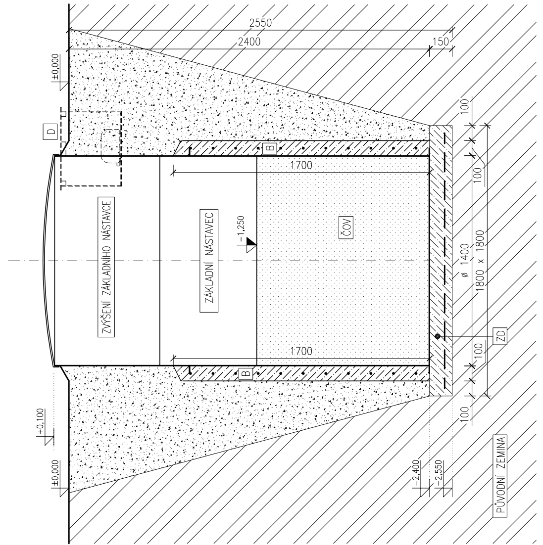
Řez
