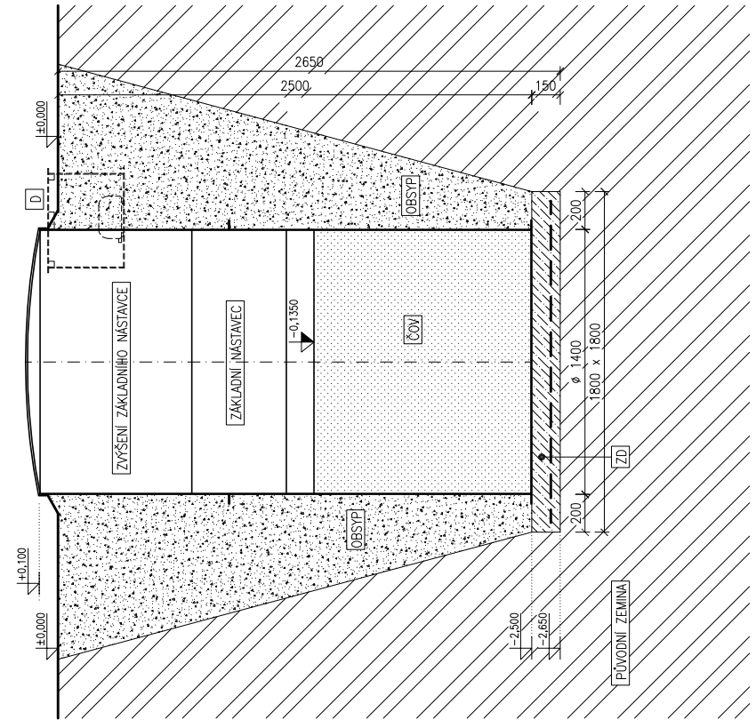
Řez
