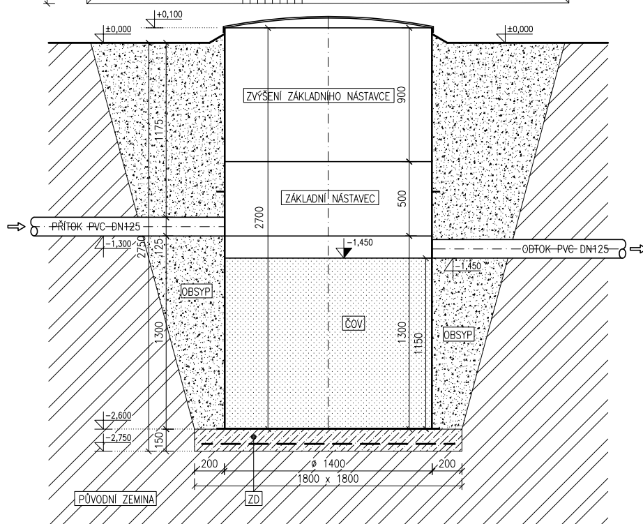
Řez
