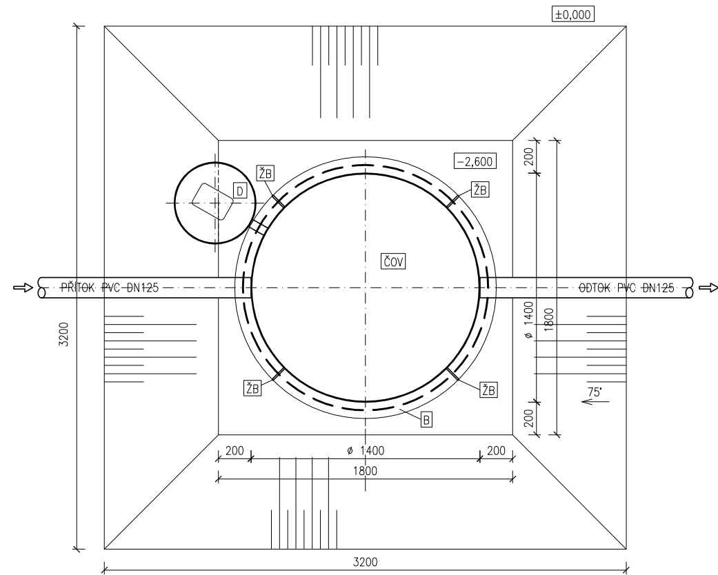
Půdorys
