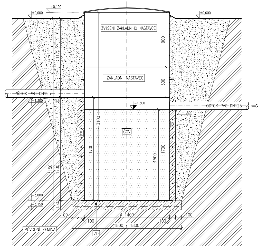
Řez
