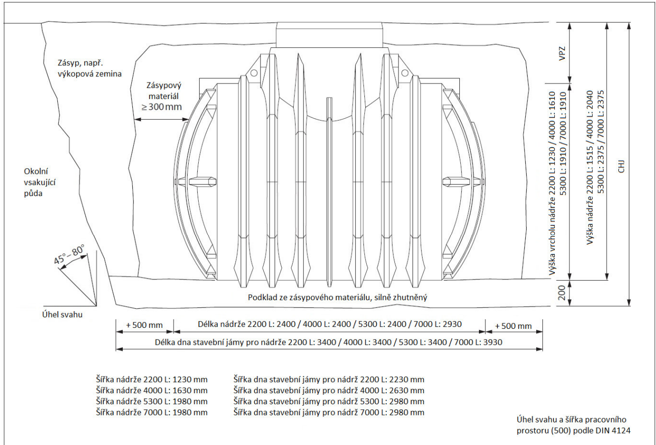
Obr. 2: Montážní velikosti
